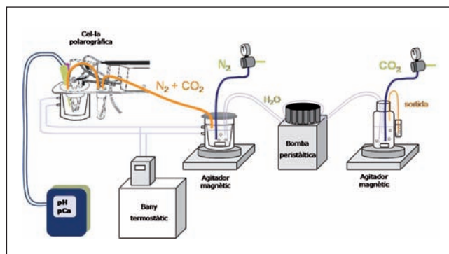
FIGURA 3. Esquema del dispositiu per ajustar el pH d'una mostra natural sense alterar-ne l'especiació tot eliminant l'oxigen amb una barreja de N_2 i CO_2 .
