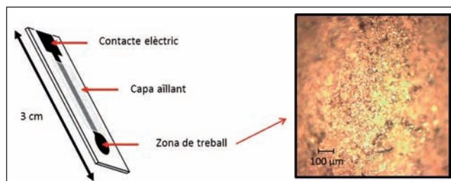
FIGURA 1. A l'esquerra, esquema d'un elèctrode serigrafat (screen printed electrode, SPE). A la dreta, imatge de la pel·lícula de mercuri dipositada a la zona de treball del SPE, fotografiada amb un microscopi òptic.
